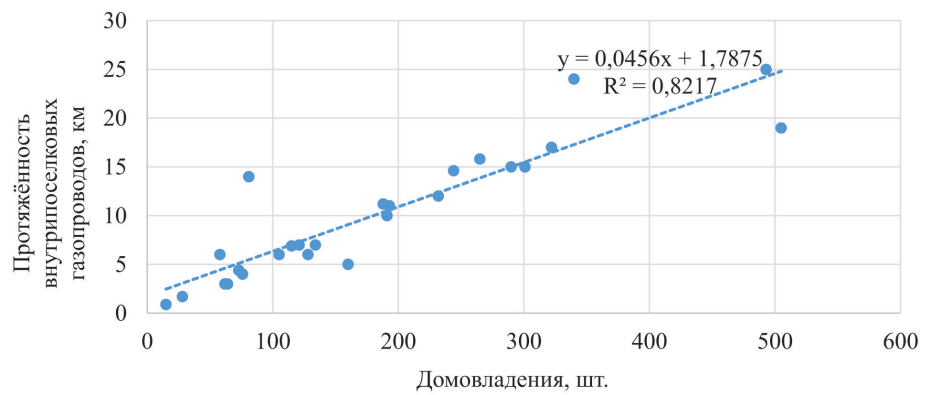
Рис. 1. Зависимость протяженности внутрипоселековых газопроводов от количества газифицированных домовладений Fig. 1. Dependence of the length of intra-village gas pipelines on the number of gasified households Источник: составлено авторами.
